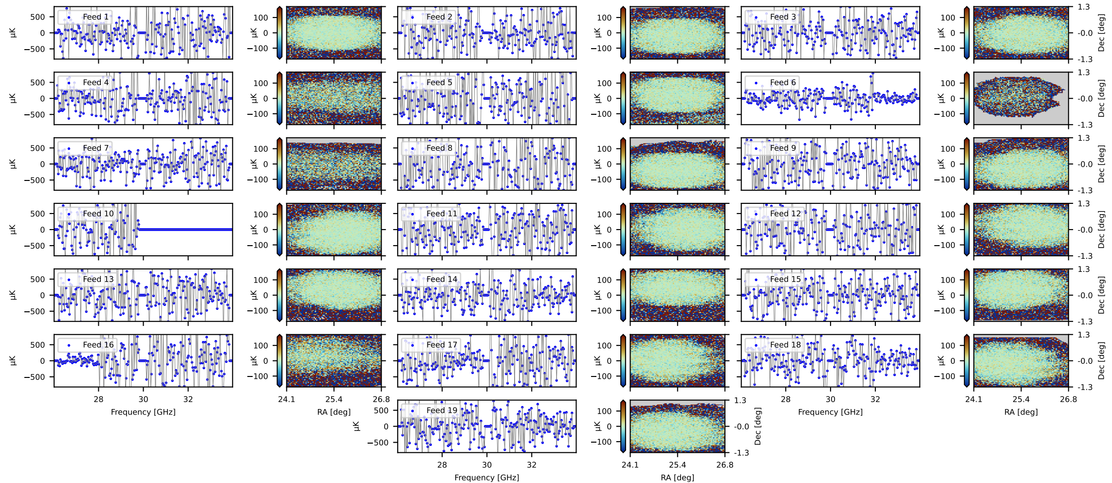
PCA mode # 4
