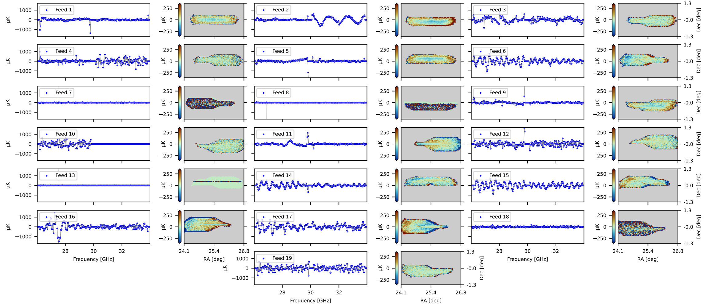
PCA mode # 0
