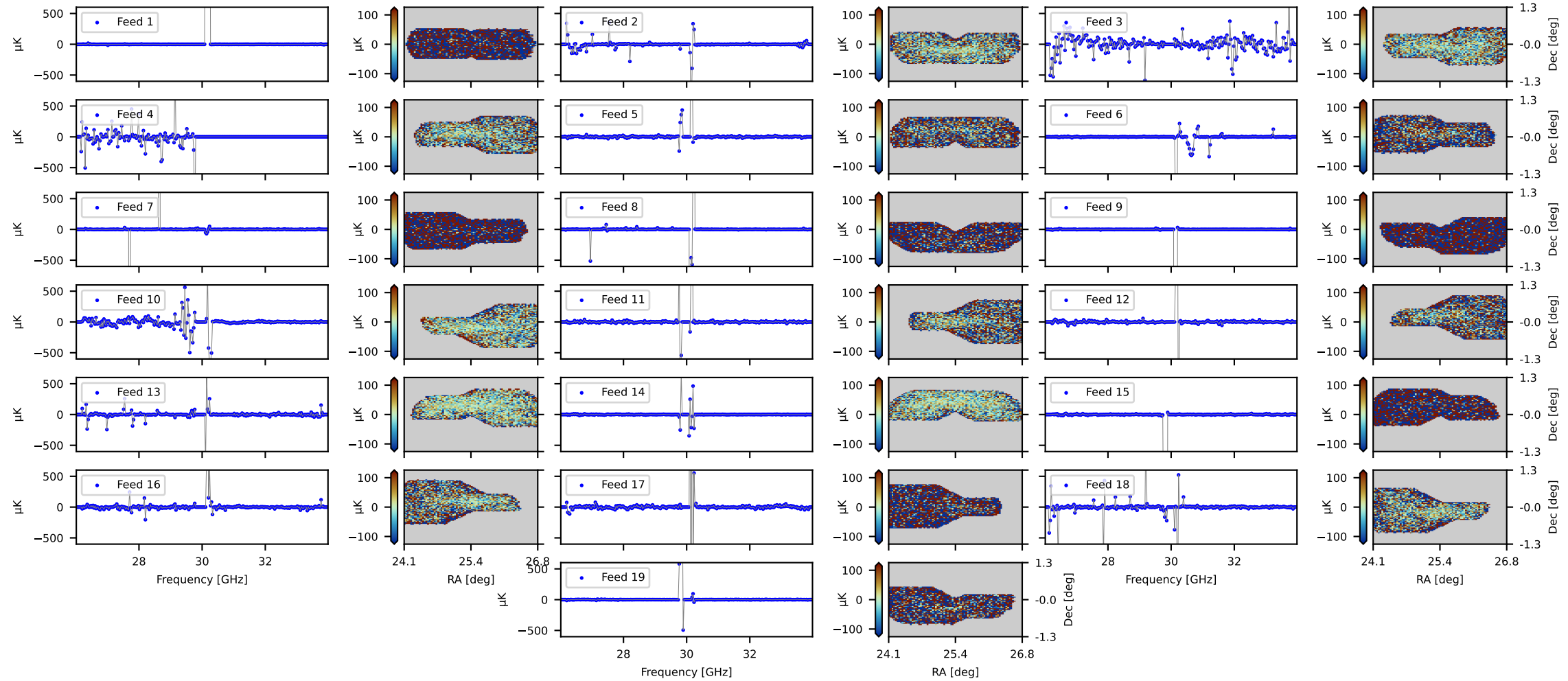
PCA mode # 2
