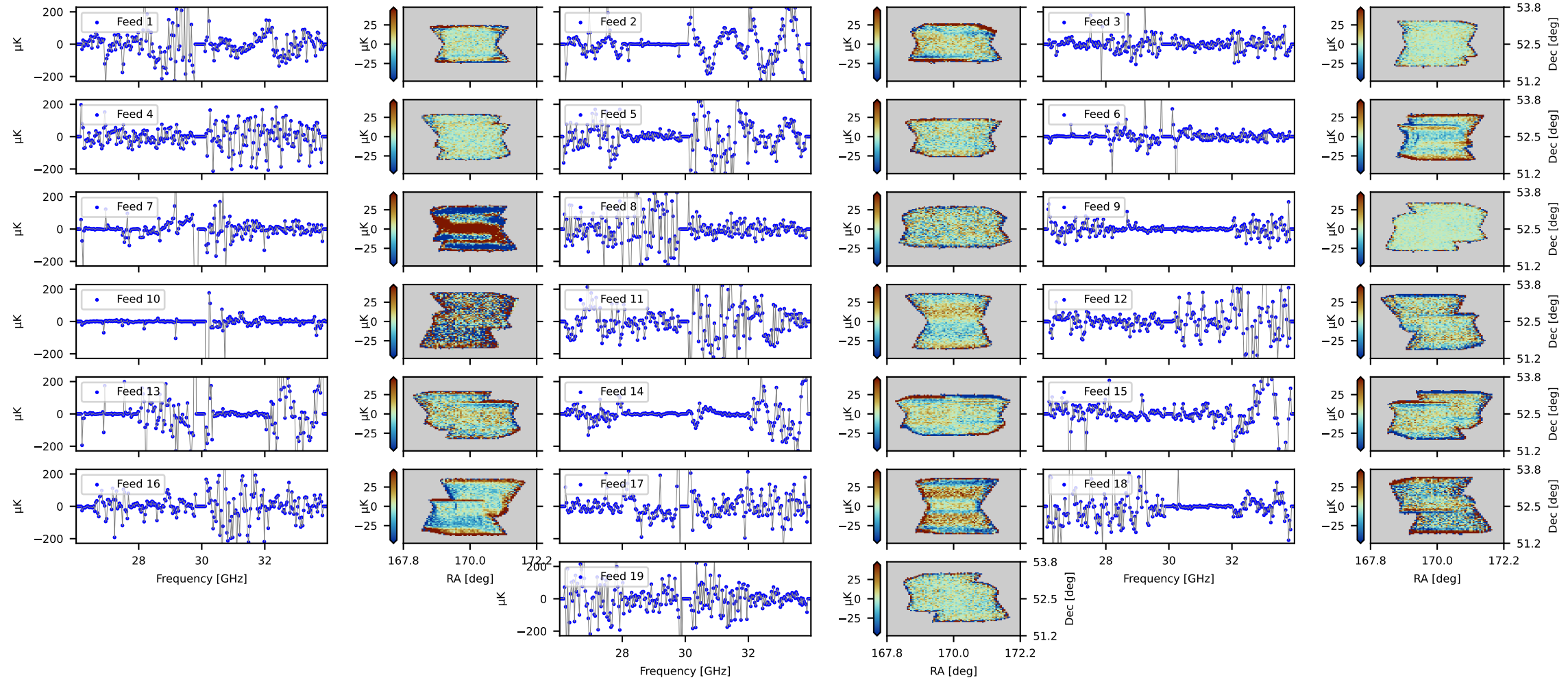
PCA mode # 2
